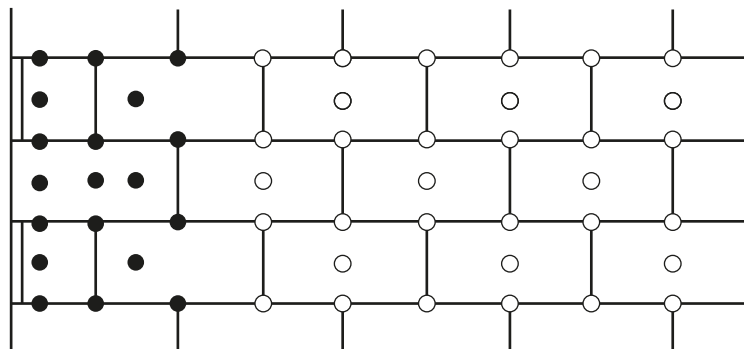
6 עוגנים/מ"ר - בקצוות 10 עוגנים/מ"ר
