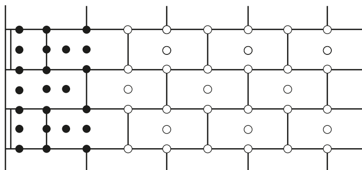
6 עוגנים/מ"ר - בקצוות 12 עוגנים/מ"ר
